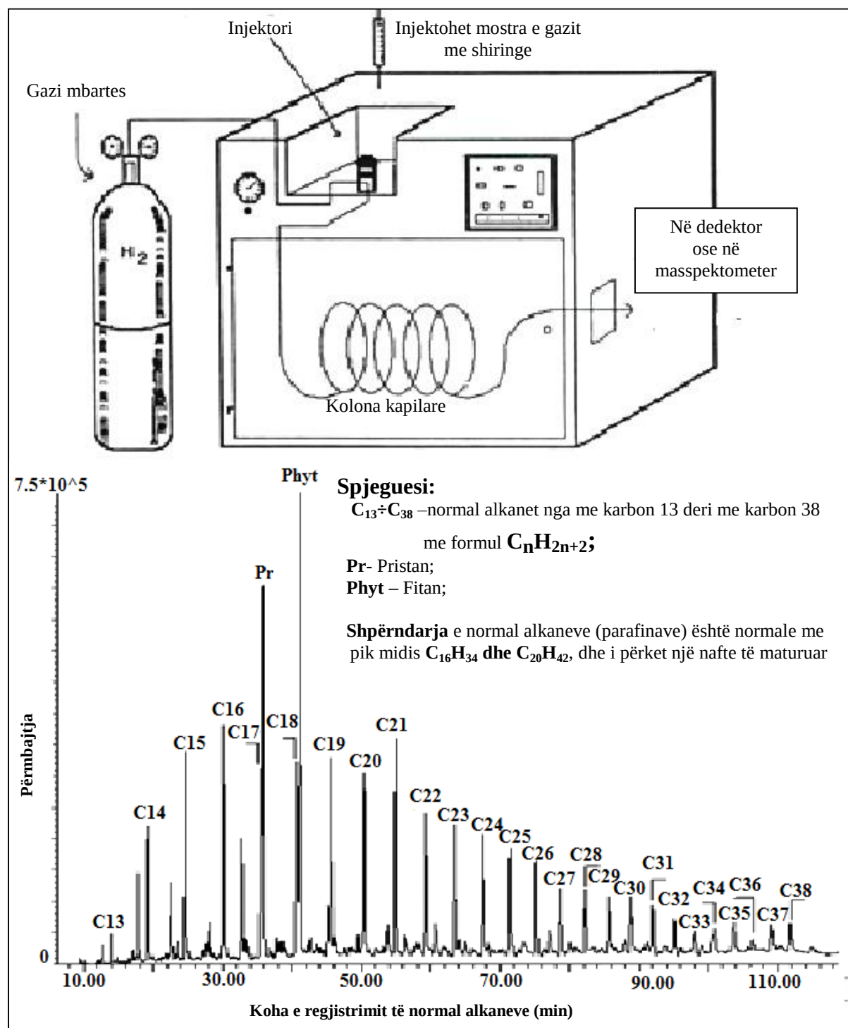
Figura 22. Skema i një gaskromatografi dhe kromatograma e një naftë të maturuar në Albanidet
