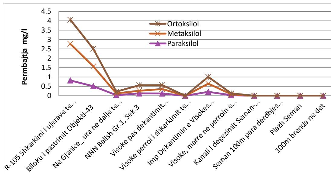
Figura 12. Përmbajtja e Ortoksilol, Metaksilol dhe Paraksilol në lumin Gjanica nga rafineria e Ballshit deri në plazhin Seman
