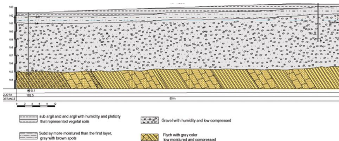
Figura 6. Profili Gjeologjik – Litologjik i zonës së rafinerisë së Ballshit (KPTHN)
