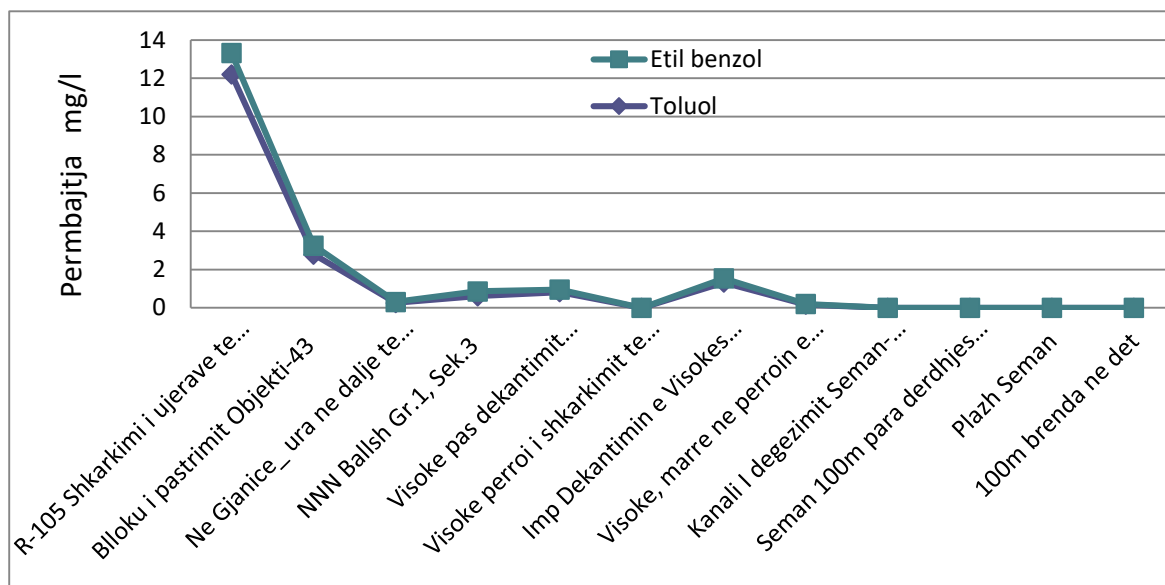
Figura 11. Përmbajtja e etil benzolit dhe tolualit në lumin Gjanica nga rafineria e Ballshit deri në plazhin Seman
