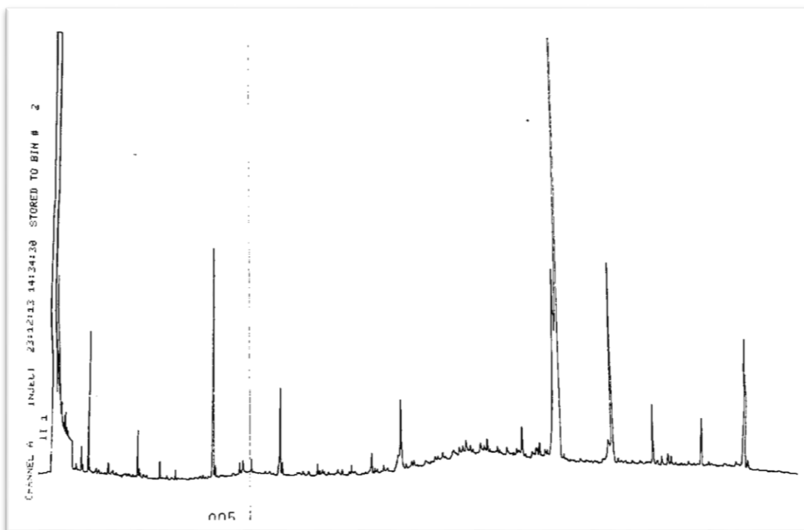
Figura 27. Kromatograma e ekstraktit të sedimentit në kampionin 4/1
