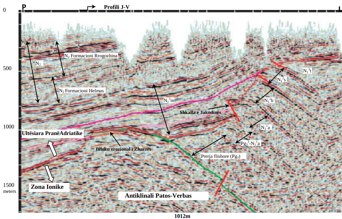
Figura 5. Profili gjeologjik në vendburimet e naftës Visok-Patos-Marinë (Prift & Dorre 2015)
