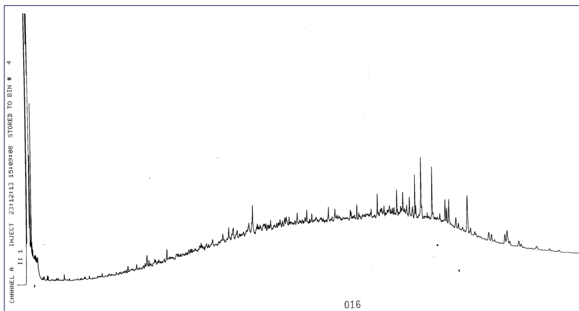
Figura 26. Kromatograma e ekstraktit të sedimentit në kampionin 3/2
