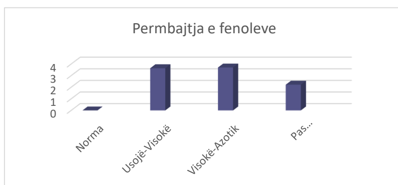
Figura 13. Përmbajtja e fenoleve në ujin e lumit Gjanicë
