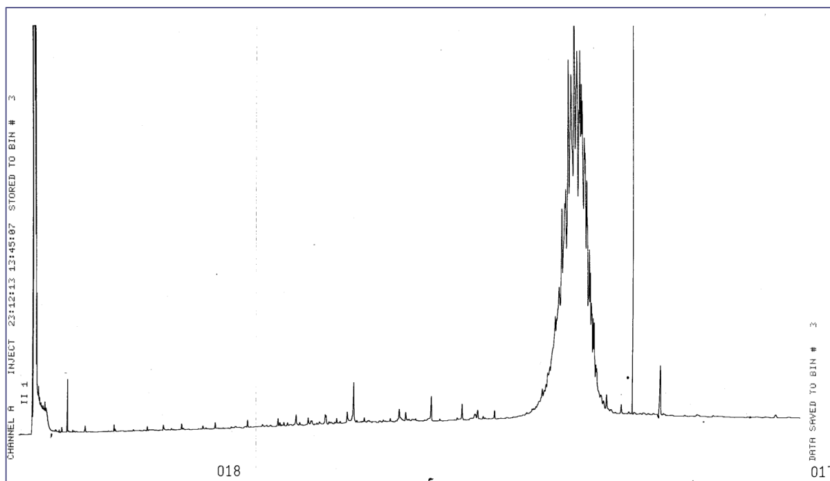
Figura 25. Kromatograma e ekstraktit të sedimentit në kampionin 2/1
