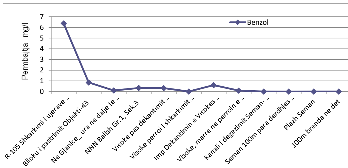
Figura 10. Përmbajtja e benzolit në lumin Gjanica nga rafineria e Ballshit deri në plazhin Seman
