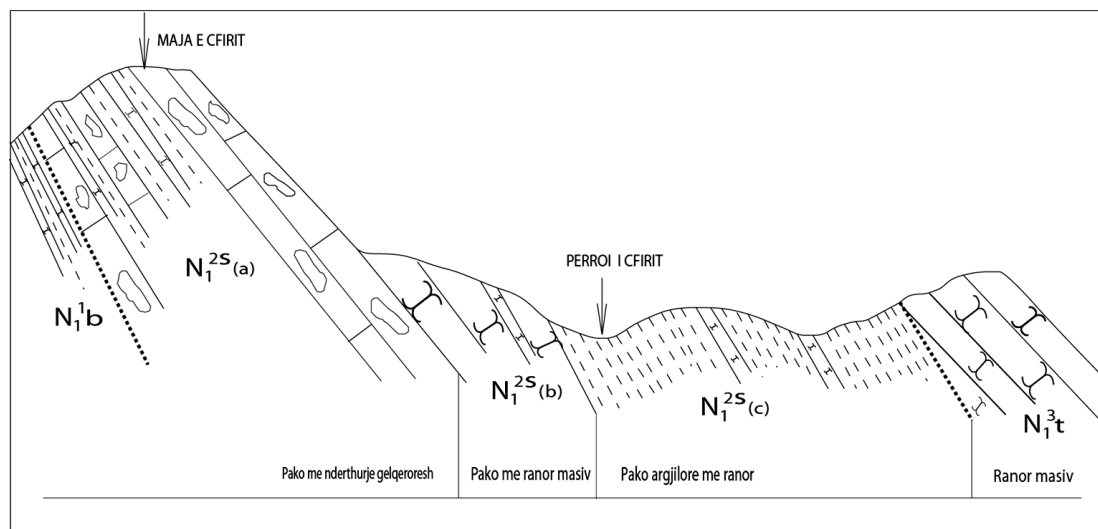
Figura 18. Depozitimet e Seravalianit transgresiv mbi ato të Burdigalianit dhe ato të Tortonianit mbi depozitimet e Seravalianit të vendosuar në mënyrë transgresive.
