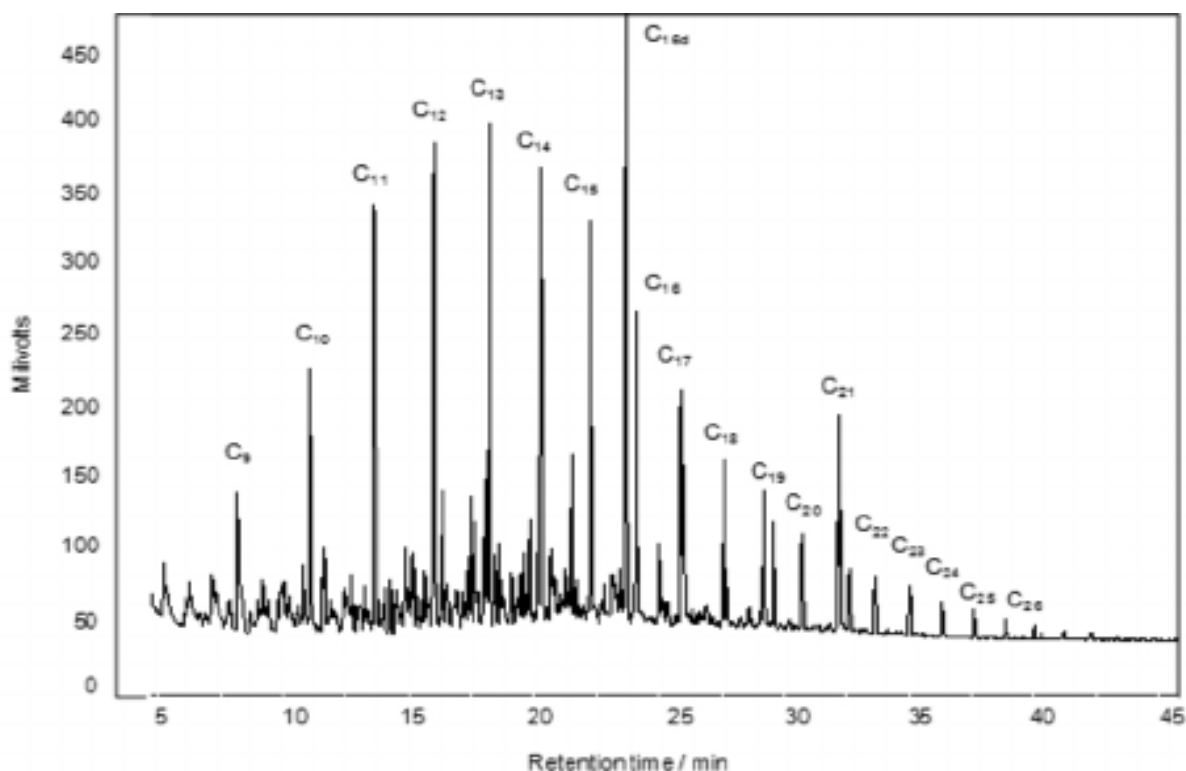
Figura 23. Kromatograma e një nafte brut në Shqipëri
