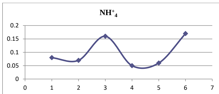
Figura 15. Vlera e \text{NH}_4 në vendmarrjet e kampionit
