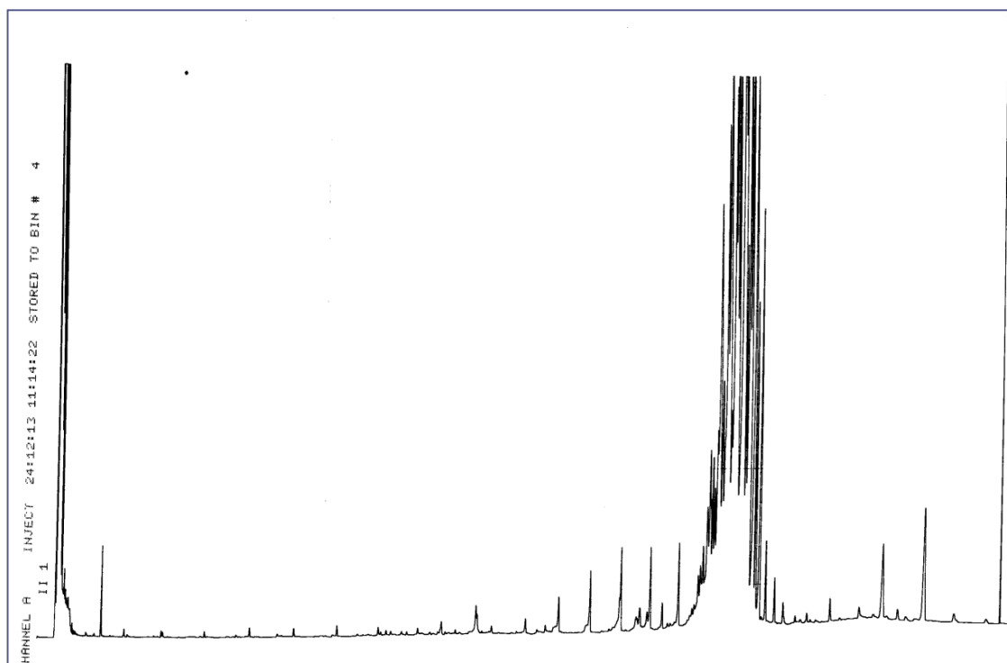
Figura 28. Kromatograma e ekstraktit të sedimentit në kampionin 4/2
