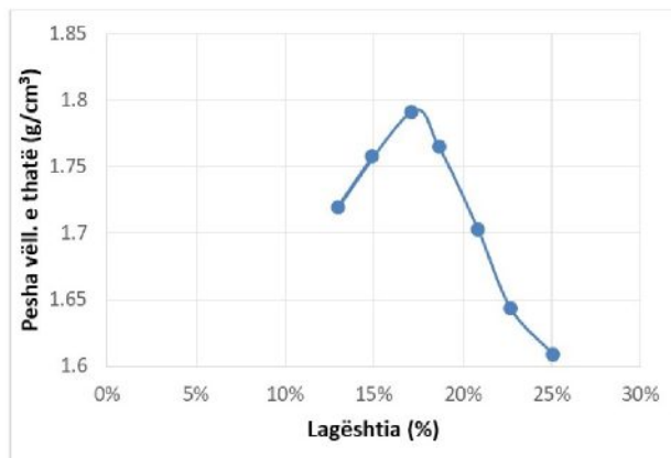
Figura 3.6: Grafiku i ngjeshmërisë për argjilën
