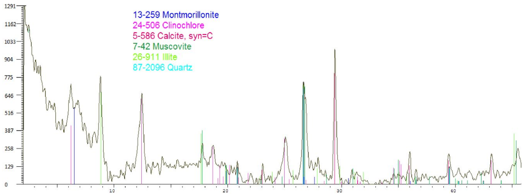
Figura 73: Prova e parë e difraksionit për argjilën
