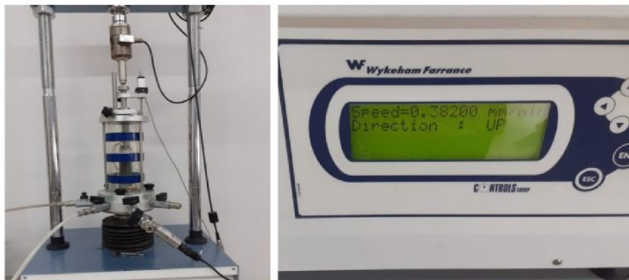
Figura 3.13: Qeliza e aparatit të triaksialit dhe shpejtësia e prerjes së kampionëve
