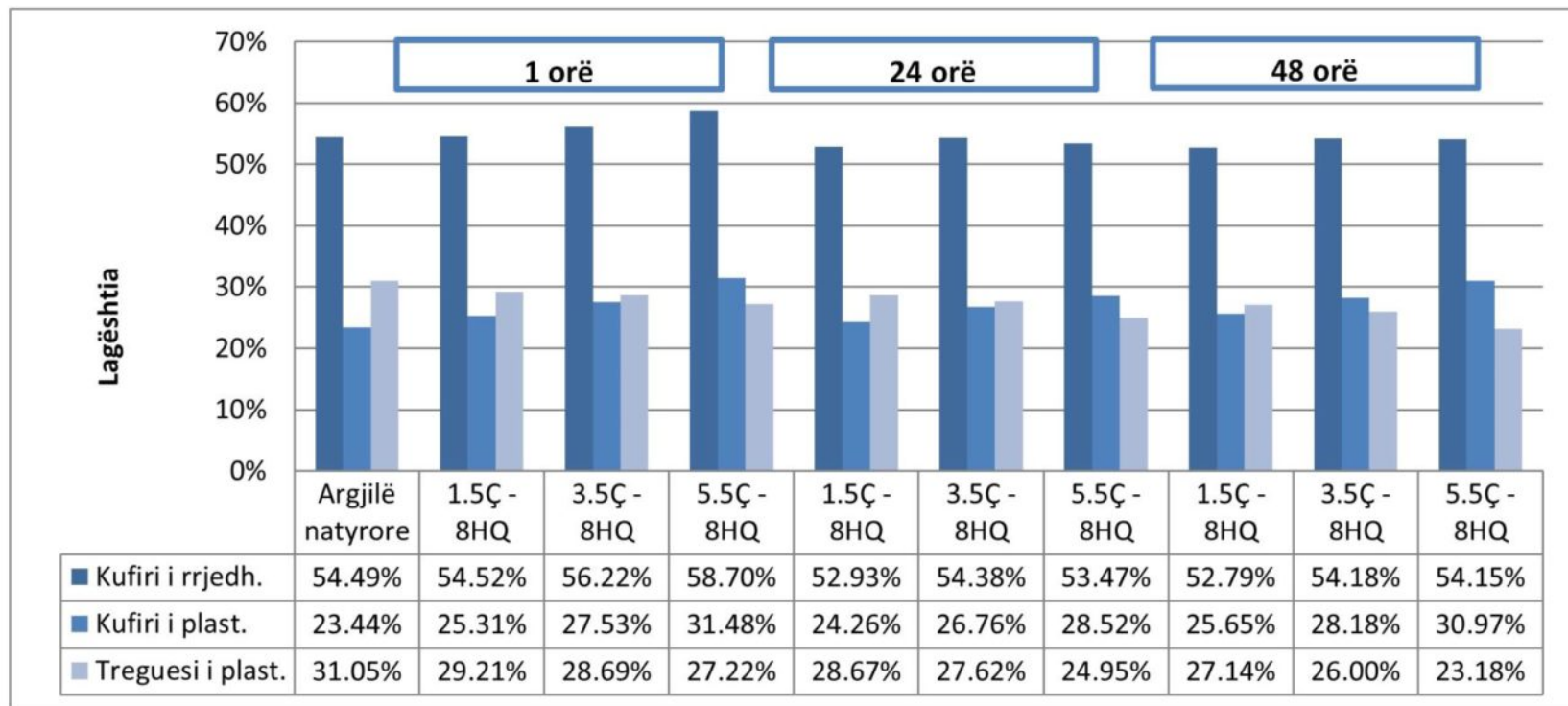
Figura 77: Ndikimi i çimentos në përzierjet me hirin qymyror
