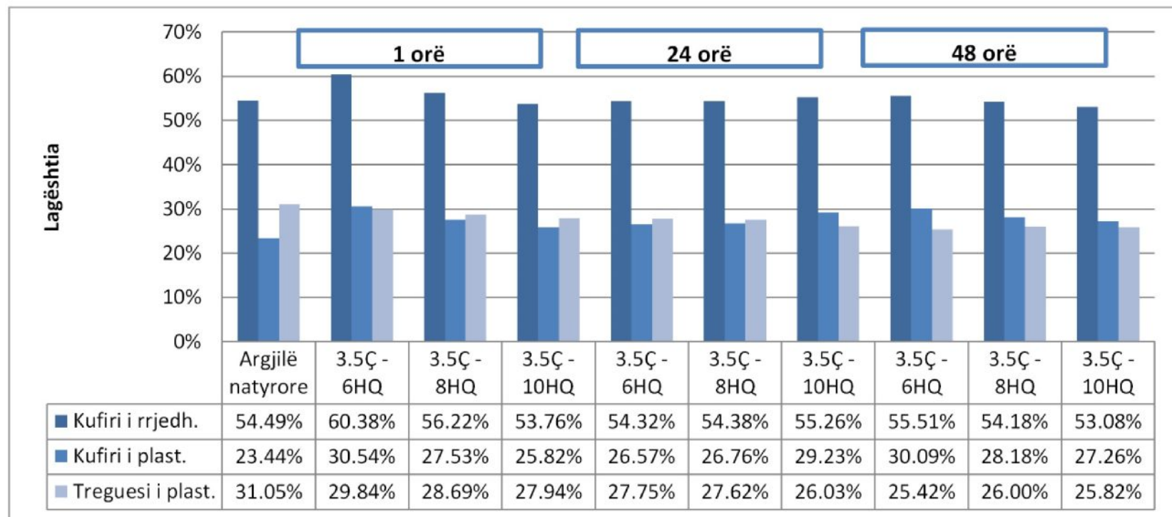
Figura 76: Ndikimi i hirit qymyror në përzierjet me çimenton
