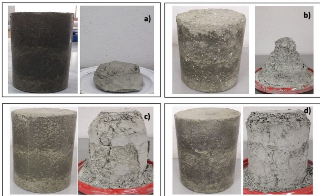
Figura 4.27: Kampionët para dhe pas ciklit të parë të lagës/tharjes a) argjilë e ngjeshur e patrajtuar, b) argjilë me 1.75% gëlqere, c) argjilë me 3% çimento dhe d) argjilë me 3.5% çimento dhe 8% hi qymyror.
