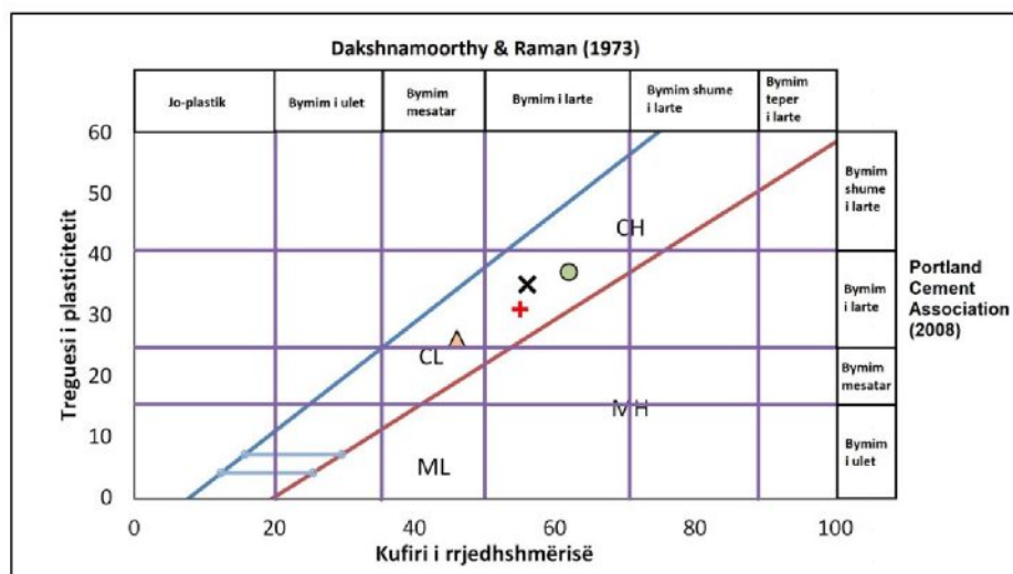
Figura 3.5: Vlerësimi i aftësisë së bymimit të argjilës së Currilave sipas skemave të propozuara nga [Dakshanamurthy & Raman, 1973] dhe [PCA, 2008]
