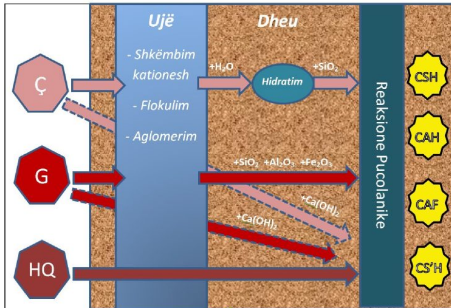
Figura 2.2: Paraqitje skematike e reaksioneve stabilizuese të çimentos, gëlqeres dhe hirit qymyror me dherat
