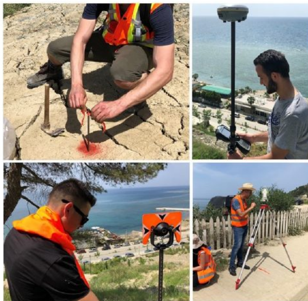
Figura 5.9: Procedura e monitorimit të shpatit përmes nguljes së piketave të hekurit dhe matjes së pikave me GPS dhe Total Station
