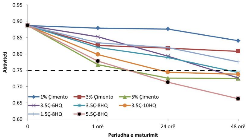
Figura 4.10: Tendenca në rënie e parametrit të Aktivitetit për sasi të ndryshme Ç/HQ
