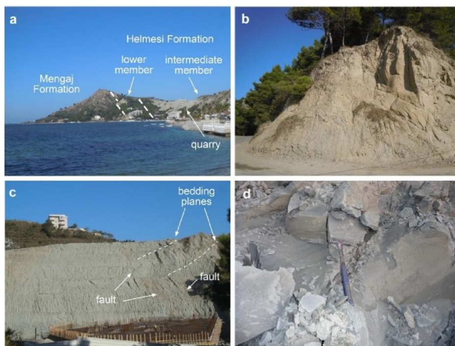
Figura 5.3: Shkëmbinjtë rrënjësorë në Durrës - a) Pamje nga plazhi i Currilave dhe e kodrës së Malit të Durrësit (187 m) nga ana jugore, me një rënie 40 gradë në lindje që janë formacionet e Maglajt dhe Helmasit (Mesinian dhe Pliocen i poshtëm, respektivisht); b) formacionet e Helmasit si përzierje rërë-argjilë; c) pamje nga gurorja e fabrikës së tullave nga drejtimi veri-perëndimor; d) argjilë e mbikonsoliduar e formacioneve të Helmasit ([Mancini et al., 2020])
