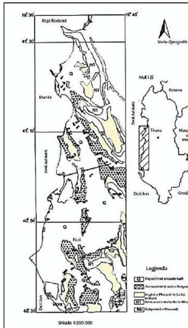
Figura 3.1: Paraqitje e shpërndarjes së formacioneve të argjilave të Pliocenit të poshtëm në Ultësirën Perëndimore (përshtatur nga [Luzati, 2017])
