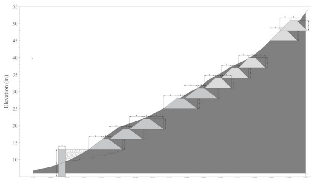
Figura 6.1: Paraqitje skematike e ndërhyrjes në kodrën e Currilave
