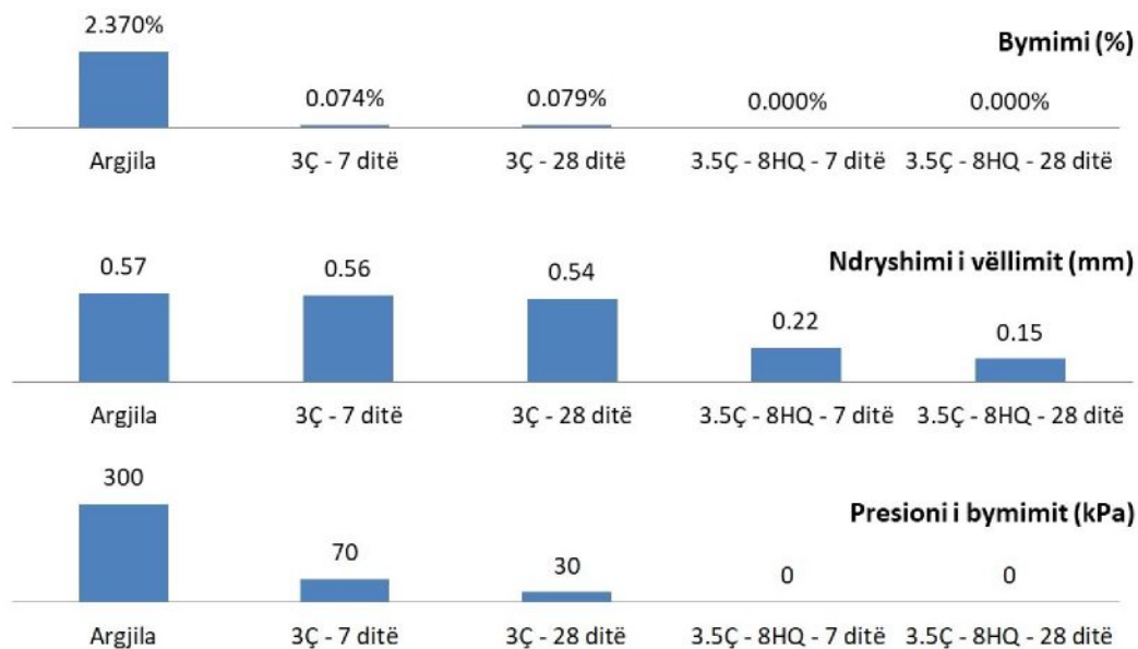
Figura 4.24: Rezultatet e provës së aftësisë së bymimit të argjilës
