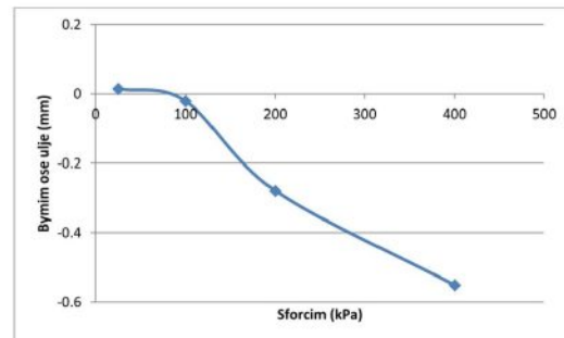
Figura 4.17: Byrimi/ulja për 3% çimento për 7 ditë
