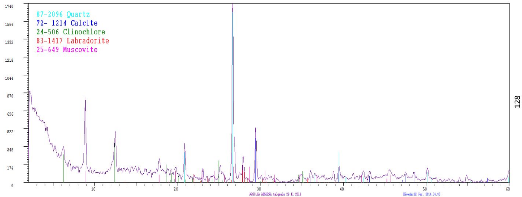
Figura 74: Prova e dytë e difraksionit për argjilën
