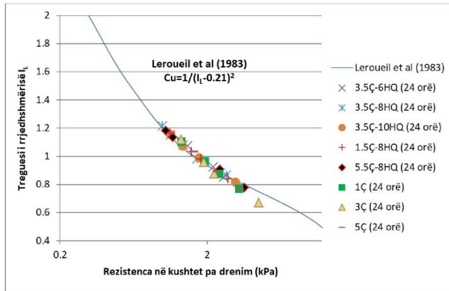
Figura 4.30: Krahasoni i vlerave të rezistencës në kushtet pa drenim sipas [Hansbo, 1957] dhe [Leroueil et al., 1983]
