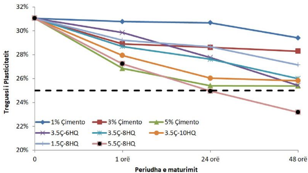
Figura 4.9: Tendencë në rënie e parametrit të treguesit të plasticitetit për sasi të ndryshme Ç/HQ
