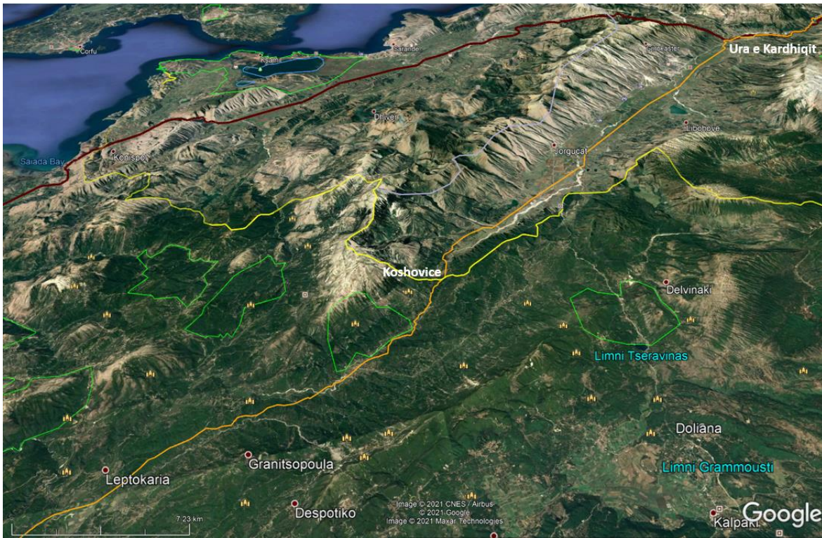
Figura 17: Paraqitje e segmentit Leptokaria (KP 51) – Ura e Kardhiqit (KP 120)
