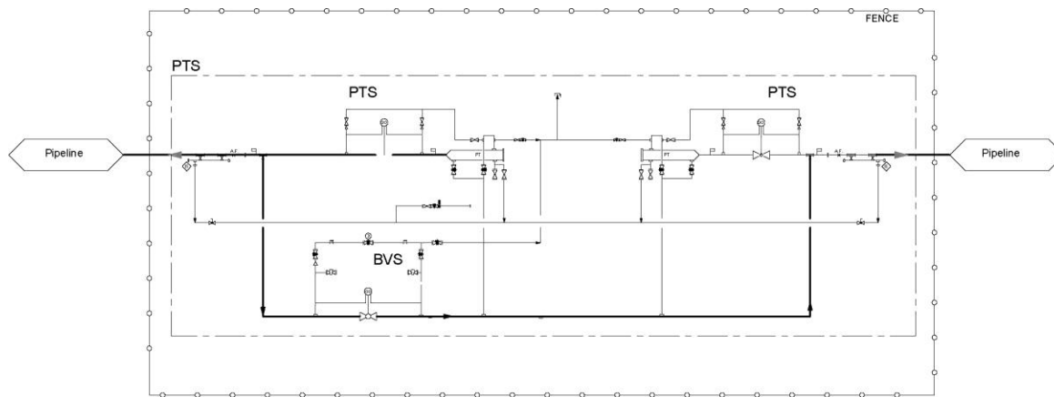
Figura 34: Konfigurimi tipik i instalimeve të lëshimit dhe mbërritjes së instrumentave të kontrollit të tubacionit (pig)
