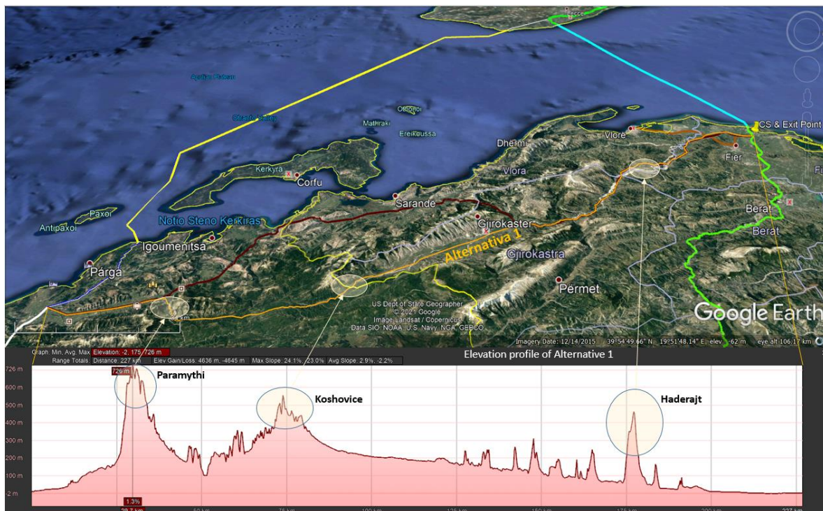
Figura 18: Profili i plotë gjatësor i Alternativës 1 së bashku me segmentet më kritike
