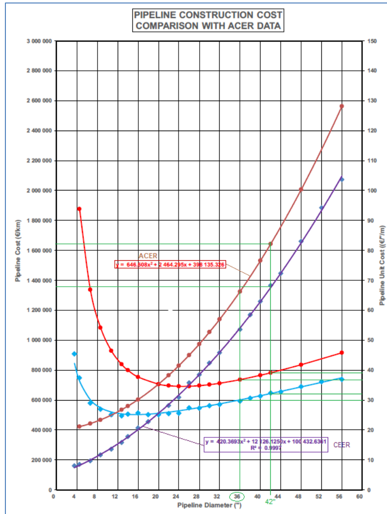
Grafiku 9: Krahاسimi i kostove të ndërtimit të tubacioneve sipas ACER dhe CEER
