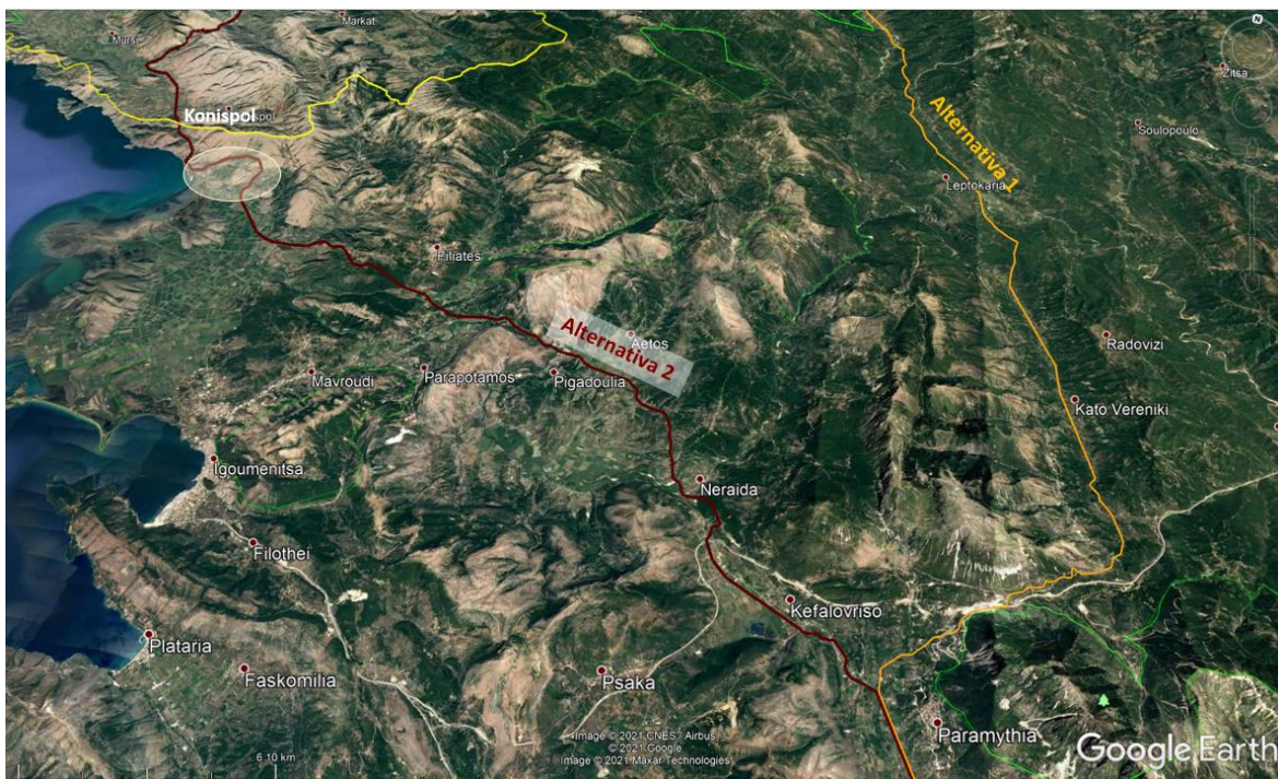
Figura 19: Alternativa 2, Segmenti Paramyithi (KP 24) – Konispol (KP 67)
