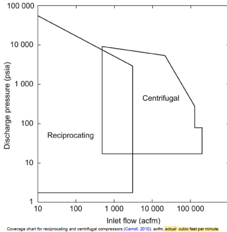
Grafiku 1: Përshtatshmëria e llojeve të pompave dhe kompresorëve në funksion të rregjimit të operacioneve
