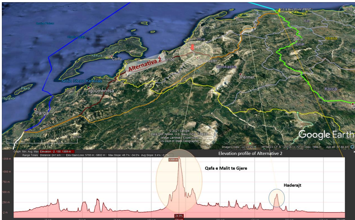
Figura 24: Profili i plotë gjatësor i Alternativës 2 së bashku me segmentet më kritike.
