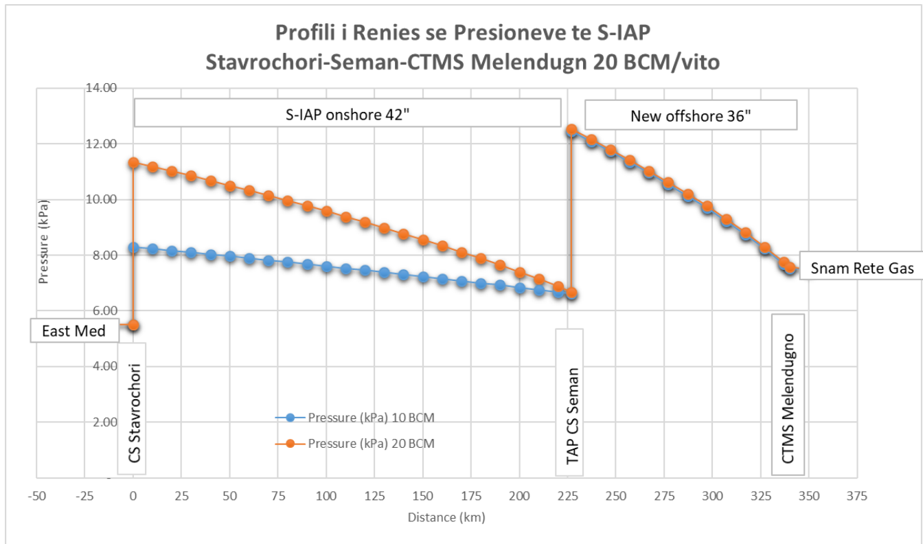
Grafiku 8: Kurba e Presioneve prej stacionit të kompresorëve në Stavrochri deri në CTMS Melendugno për regjimet 10 BCM/vit dhe 20 BCM/vit
